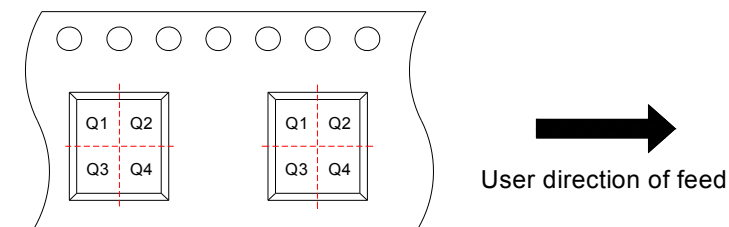
Pin 1 quadrant:Q1
