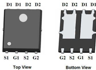
PDFN5X6-8L(Dual)
