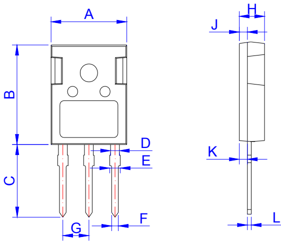
TO-247J
