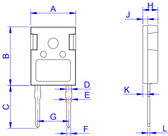
TO-247J-2L
