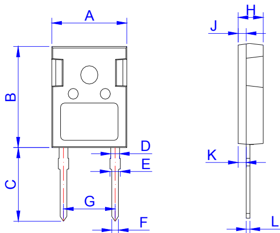
TO-247J-2L
