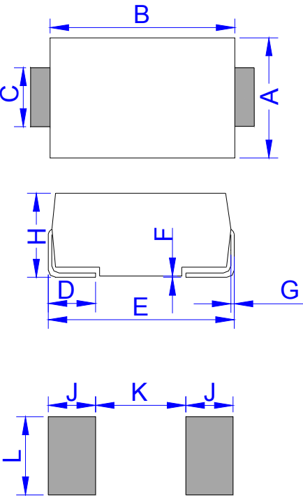
DO-214AC (SMA)
